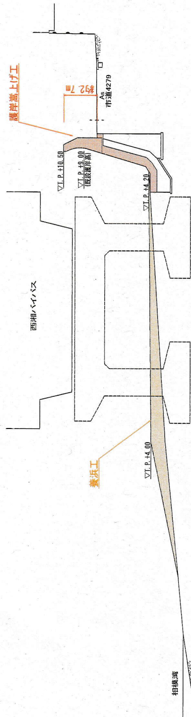
標準横断面図
